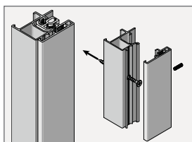
Tvådelad sidokanal 38 x 31 mm
