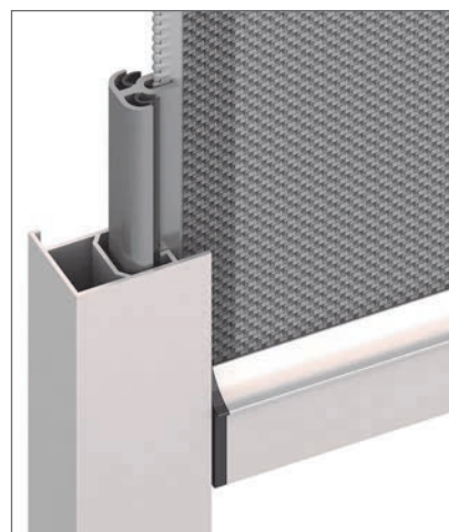
Underlist 24 x 39 mm, samt zipfunktion
