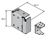
Endebeslag 50/70 mm incl U-beslag til midtplacering.
