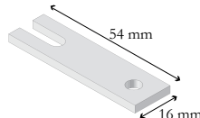
Afstandsstykke til loftbeslag 50/70 mm, kædetræk/motor
