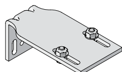
Forskydelig vinkel, 4-6 cm 16/25 mm
