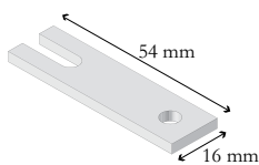
Avstandstykke til takmontering - kjedetrekk/motor (standardbeslag)
