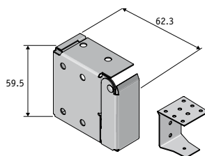
Endebeslag, spesial - U-beslag til midtplassering
