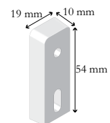
Avstandstykke, 10 mm til 70 mm
