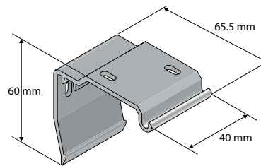
Design XL, klipsbeslag
