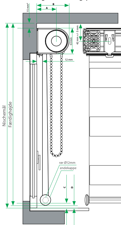
Væg – monteringsprofil
