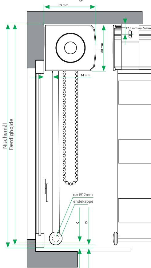
Loft/væg – kassette
