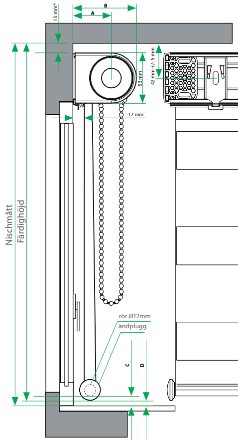
Vägg – monteringsprofil
